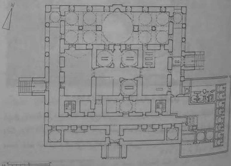
مخطط للمدرسة الأشرفية الكبرى
